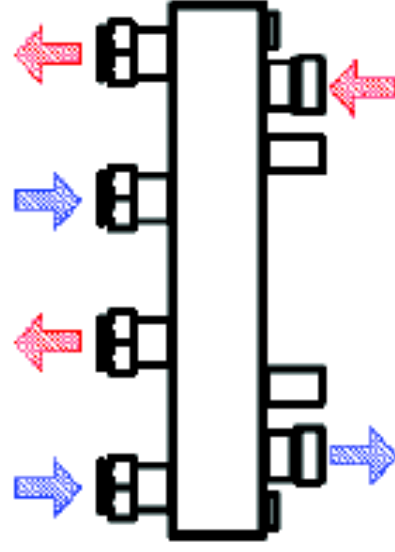
Hidravlična kretnica + 2 veji
