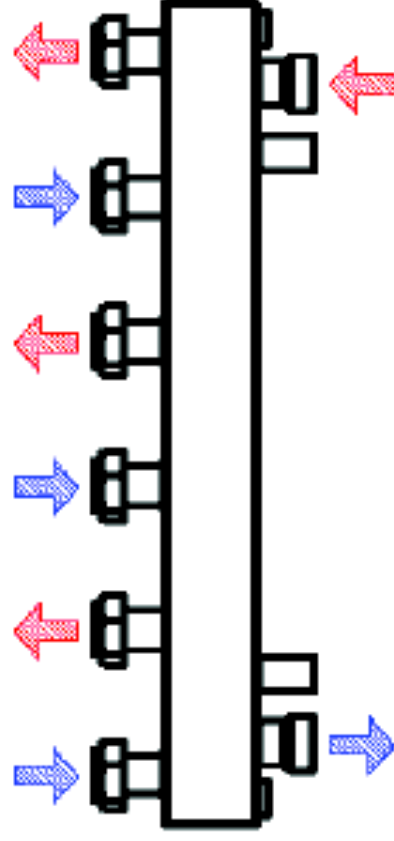
Hidravlična kretnica + 3 veje
