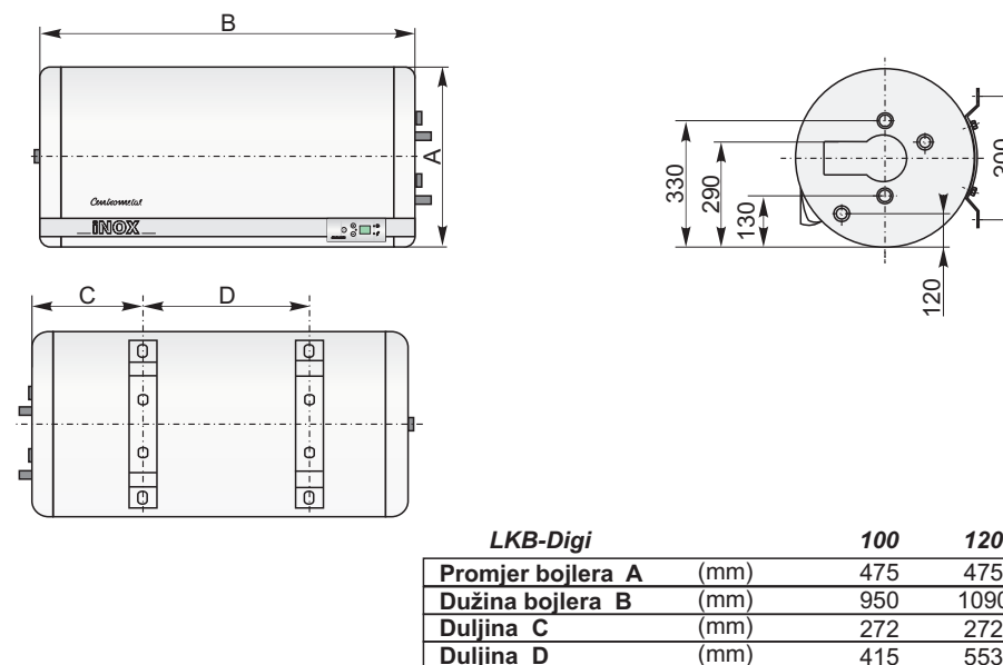
Slika 2. - Osnovne dimenzije kombiniranok bojlera SKB-Digi (desna izvedba)
