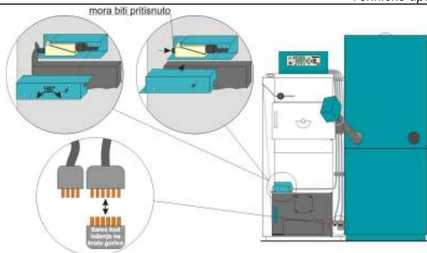
Loženje kotla krutim gorivom
